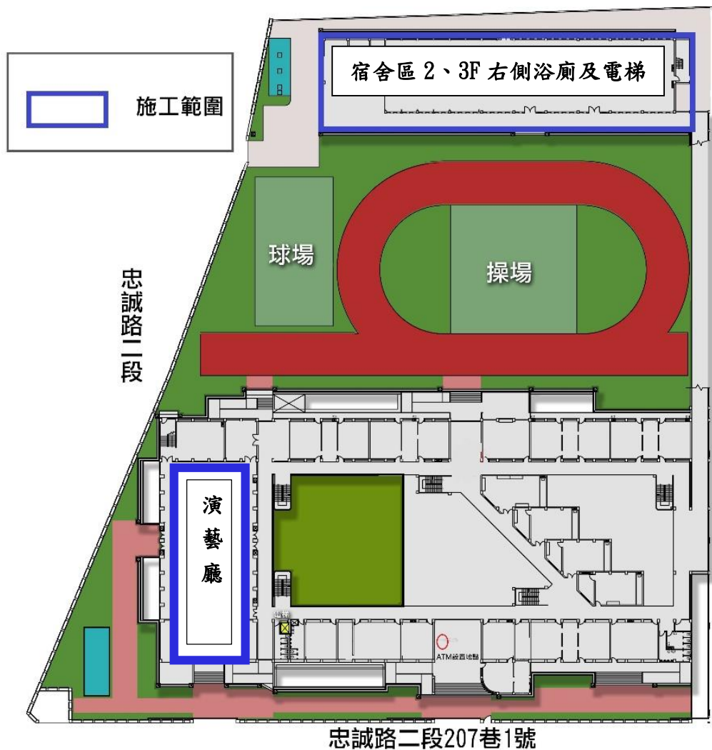
臺北市立啟明學校 8~9 月施工範圍圖 一樓演藝廳及宿舍 2、3F 右側浴廁及無障礙電梯 (111 年 8 月 2 日開工，預計 111 年 9 月 30 日完工)
